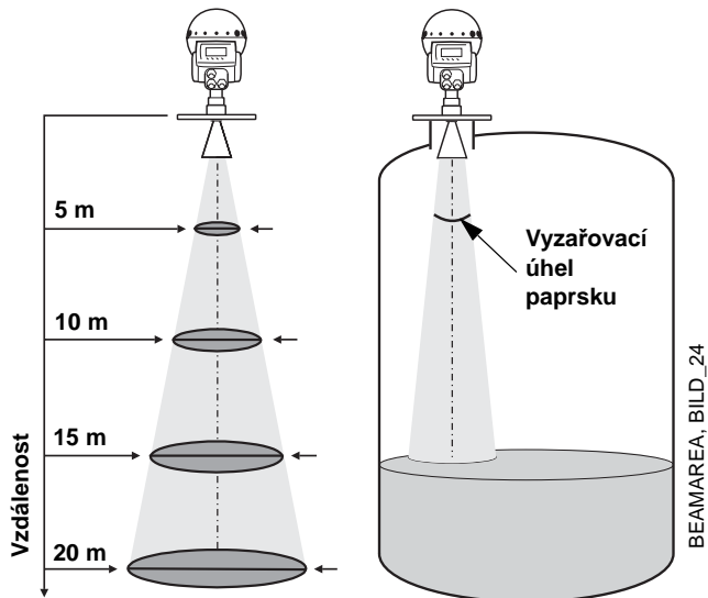
Obrázek 4. Vyzařovací úhel snímače Rosemount 5600
