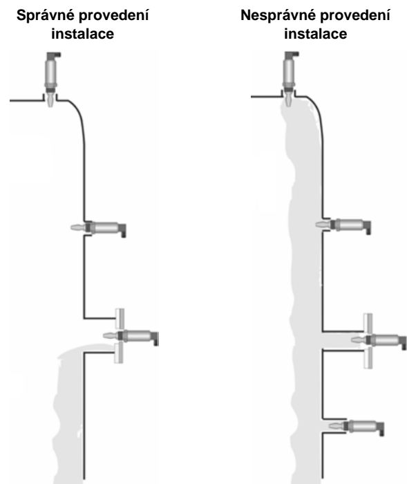
Obrázek 1. Příklady správné a nesprávné instalace spínače na nádrži
